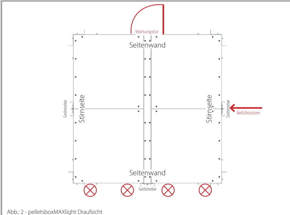
Abb.: 2 - pelletsboxMAXlight Draufsicht
